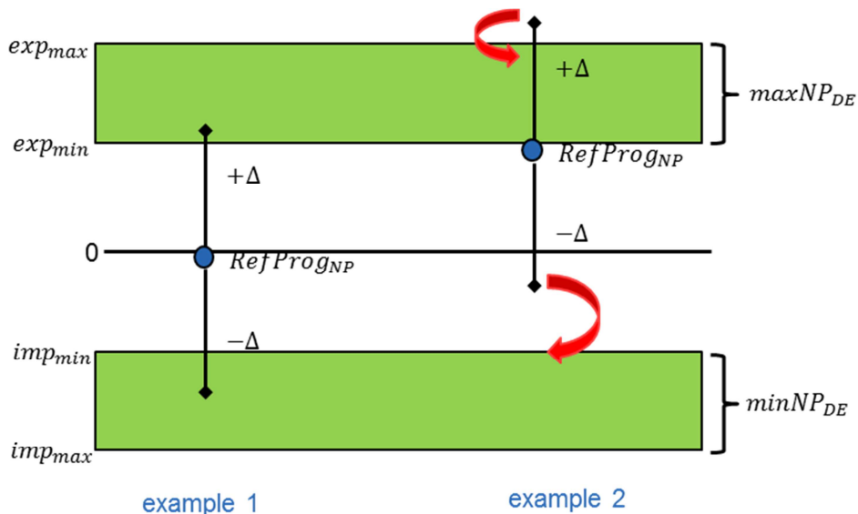
Abbildung: Ermittlung der Export- und Importbegrenzungen
